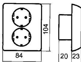
Målskisse
