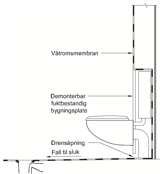
Fig. 3 Prinsippskisse – Installering i våtrom
