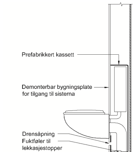
Fig. 4 Prinsippskisse – Installering i tørre rom
