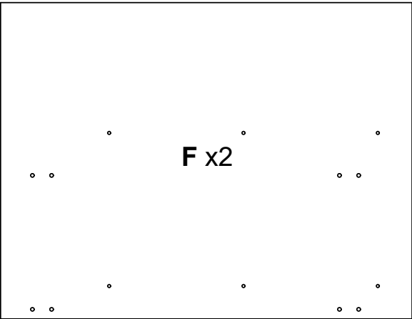
686x529x15mm
