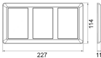
Målskisse
