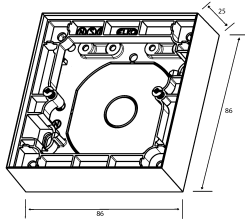
Målskisse
