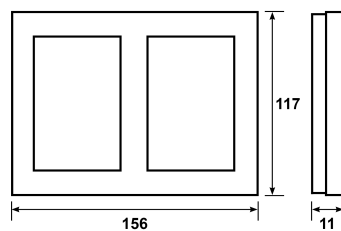
Målskisse
