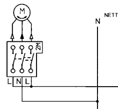
Koblingsskjema
