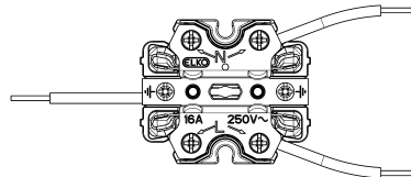
Koblingskjema
