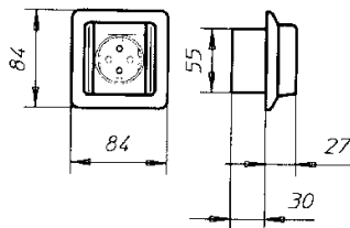
Målskisse
