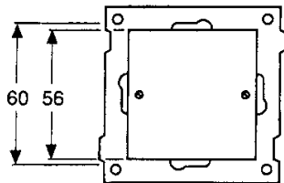
Målskisse
