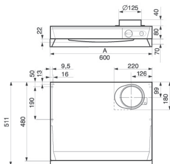
Målskisse
