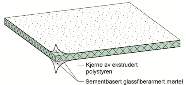
Fig. 1 Oppbygningen av Tetti Våtromsplate. Platen er symmetriske med armert mørtel på begge sider
